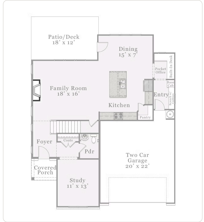
OPTIONAL - FIREPLACE
